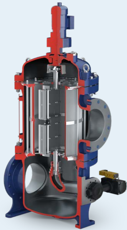
Feinsiebzylindereinsatz
