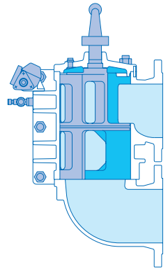
旋塞阀切换装置
